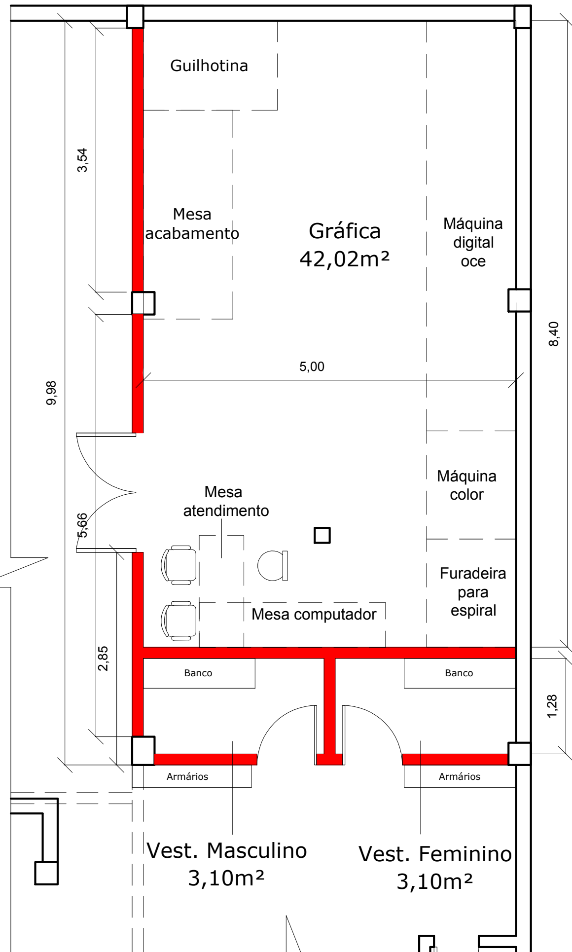
PLANTA BAIXA TÉRREO ESCALA 1:50
