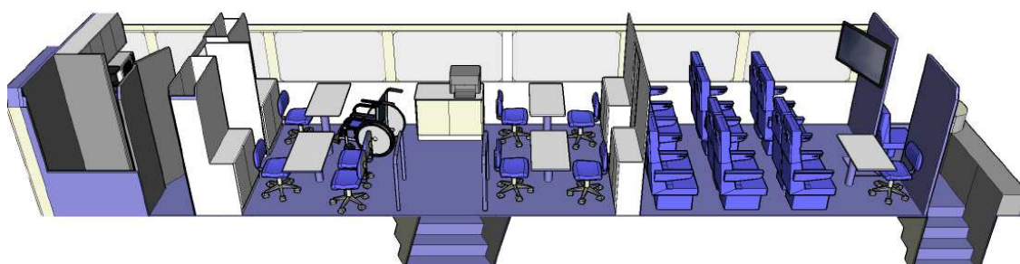
PERSPECTIVA GERAL
